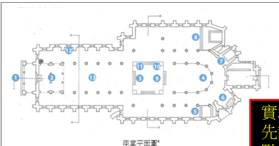
座堂平面圖 4
